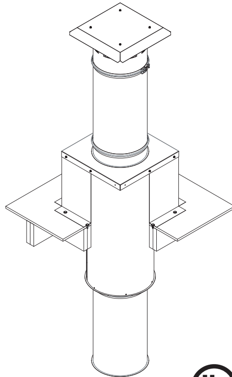
Chimney
